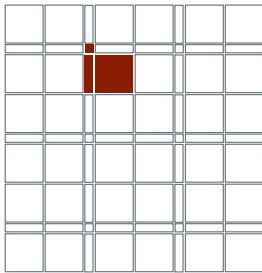
cuadrada 33 x 33 x 1,8 cm tira 33 x 7 x 5 cm dot 7 x 7 x 1,5 cm
