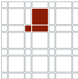
cuadrada 41 x 41 x 2,3 cm tira 15 x 41 x 2,3 cm dot 15 x 15 x 2,3 cm
